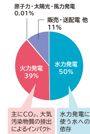
●図3. エコロジカル・フットプリントの算定結果
