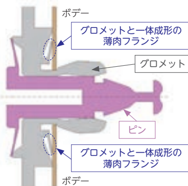
【締結部 本製品構造】
