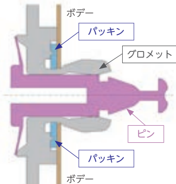
【締結部 従来構造】
